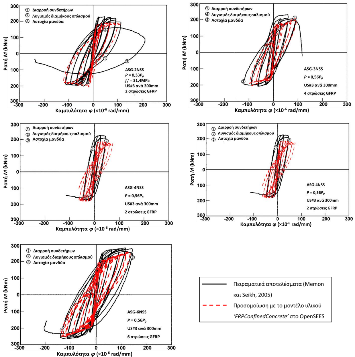
Σχήμα 2: Σύγκριση αποτελεσμάτων προσομοίωσης με αντίστοιχα πειραματικά σε τετραγωνικά υποστυλώματα οπλισμένου σκυροδέματος ενισχυμένων με GFRP υπό ανακυκλιζόμενη φόρτιση [6].
